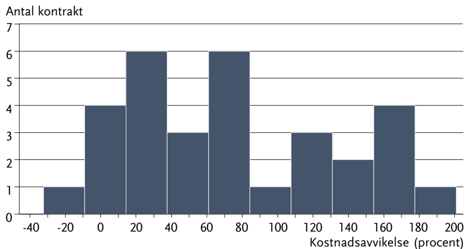
Figur 1 Fördelning av kostnadsavvikelser: hela kontraktet
